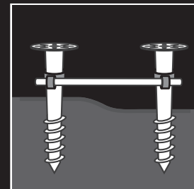
スクリー杭の横揺れ 防止に
