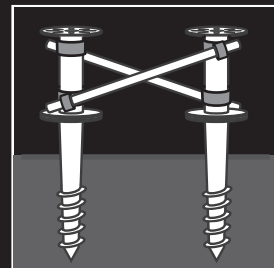
ダブルフランジを使用した 場合の補強に
